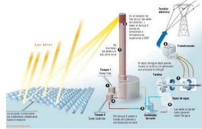
Centrales Termosolares
